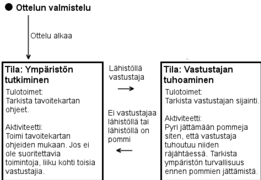
KUVIO 30 Videopeliin toteutettu tilakone
