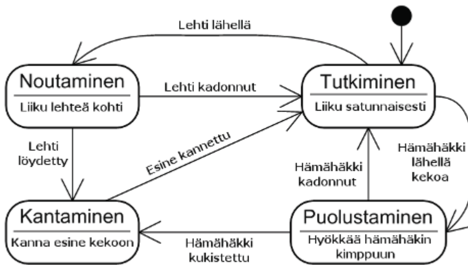
KUVIO 12 Esimerkki tilakoneen käytöstä
