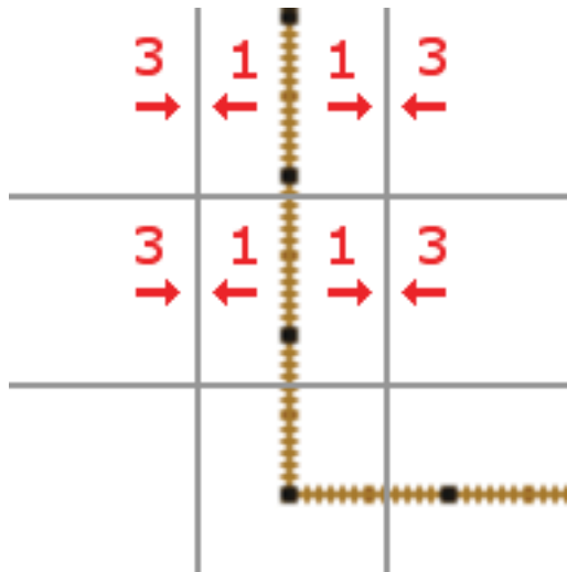
KUVIO 4 Esimerkki painotetusta suunnatusta graafista
