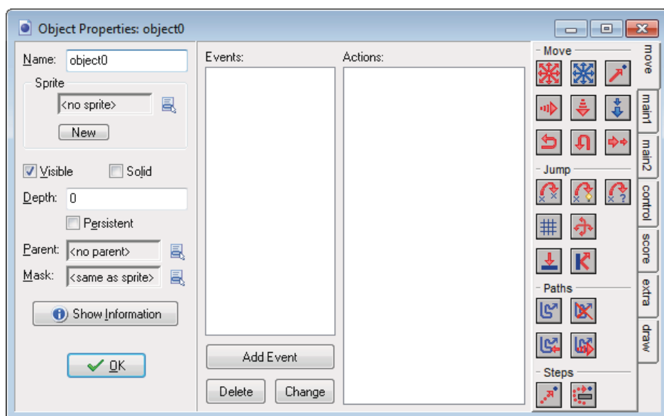
KUVIO 16 Game Maker 8 -ohjelman objektieditorin käyttöliittymä
