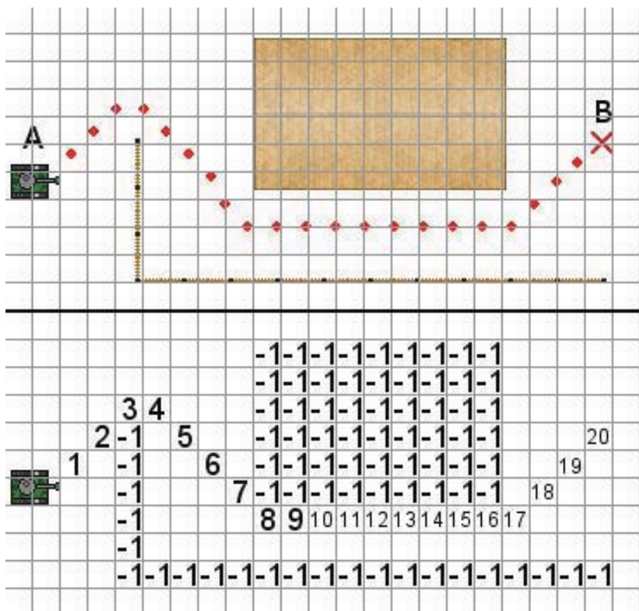
KUVIO 13 Esimerkki tavoitekartasta
